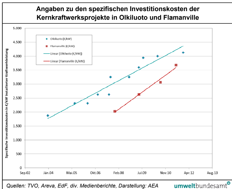
Abbildung 6: Angaben zu den spezifischen Investitionskosten der Kernkraftwerksprojekte in Olkiluoto und Flamanville, die zwischen 2004 und 2012 veröffentlicht wurden.
