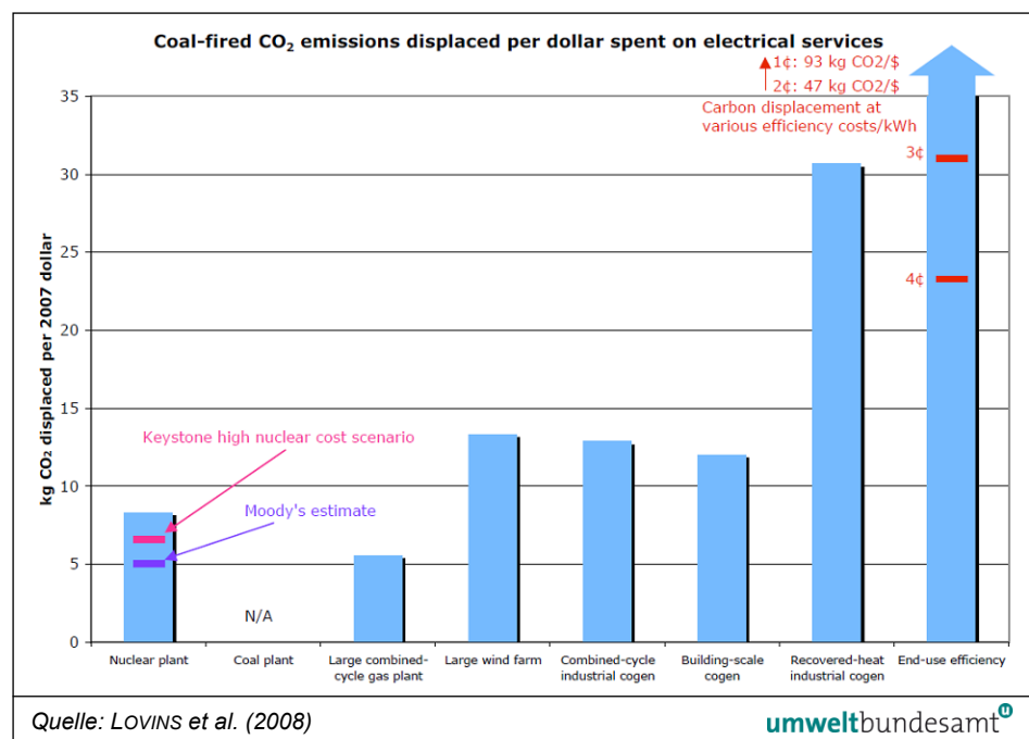
Abbildung 8: Darstellung der Vermeidung von CO 2 -Emissionen beim Ersatz von Kohlekraftwerken durch andere Technologien in kg vermiedene CO 2 -Emissionen je investiertem USD.
