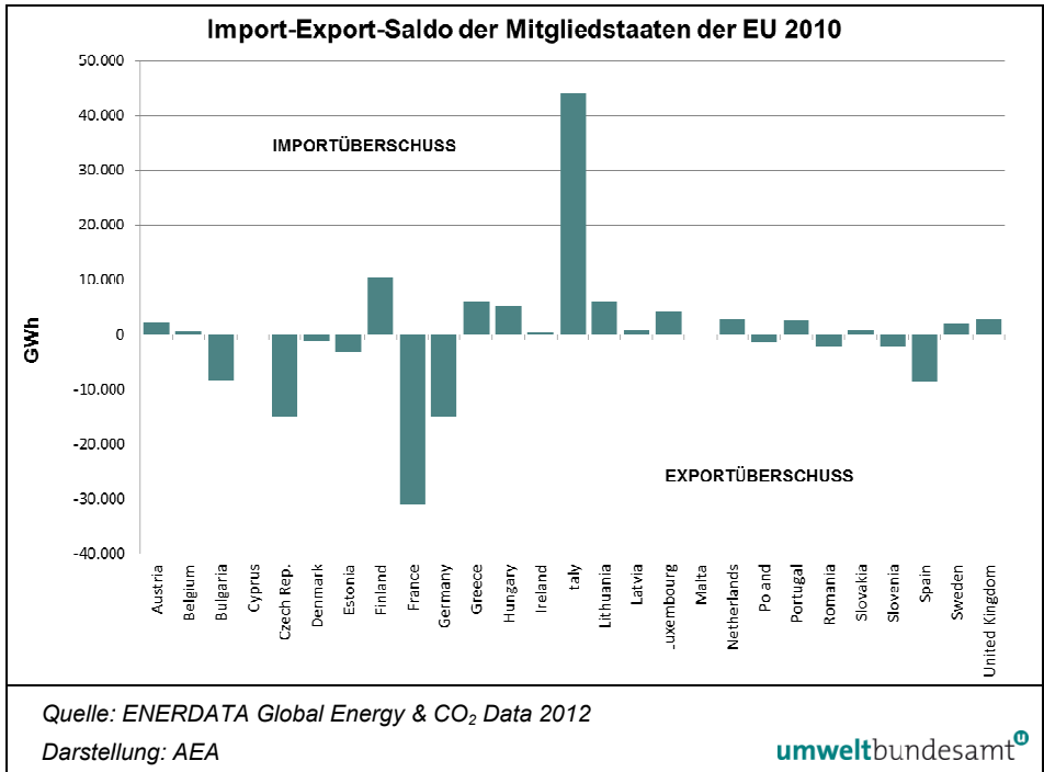
Abbildung 1: Strom-Import-Export-Saldo der EU-Mitgliedstaaten 2010:
