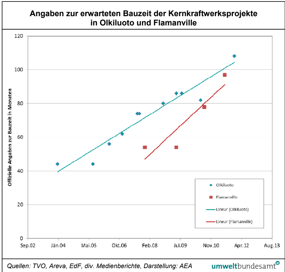
Abbildung 7: Angaben zur erwarteten Bauzeit der Kernkraftwerksprojekte in Olkiluoto und Flamanville, die zwischen 2004 und 2012 veröffentlicht wurden.
