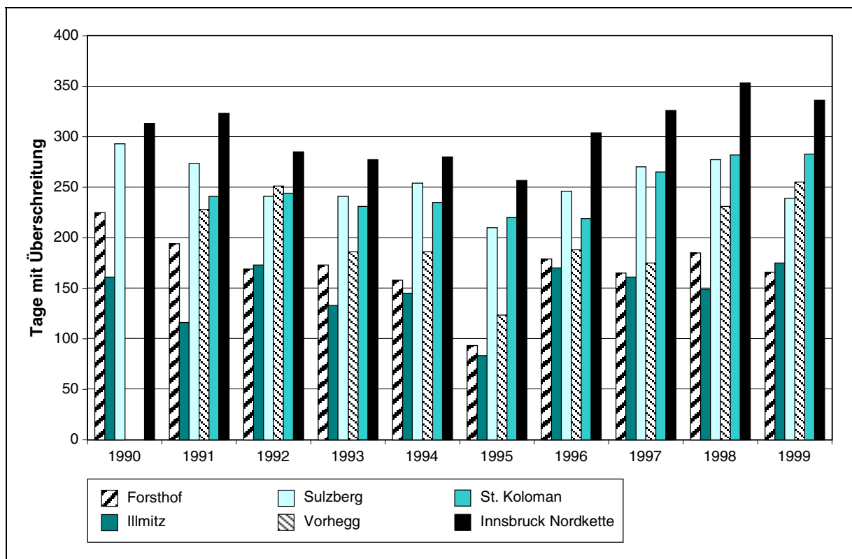
Abb. 12: Anzahl der Tage mit Überschreitung des Tagesmittelwertes von 0,065 \text{ mg/m}^3 an ausgewählten Messstellen.
