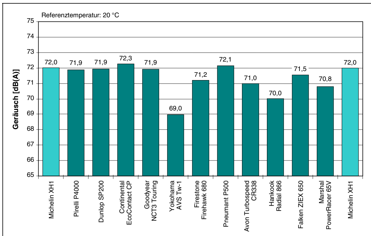
Abb. 6b: Schallpegel von Reifen verschiedener Erzeugung, gemessen nach Vorschlag zur Richtlinie 92/23/EWG. Reifen: 195/65 R 15 91V.
