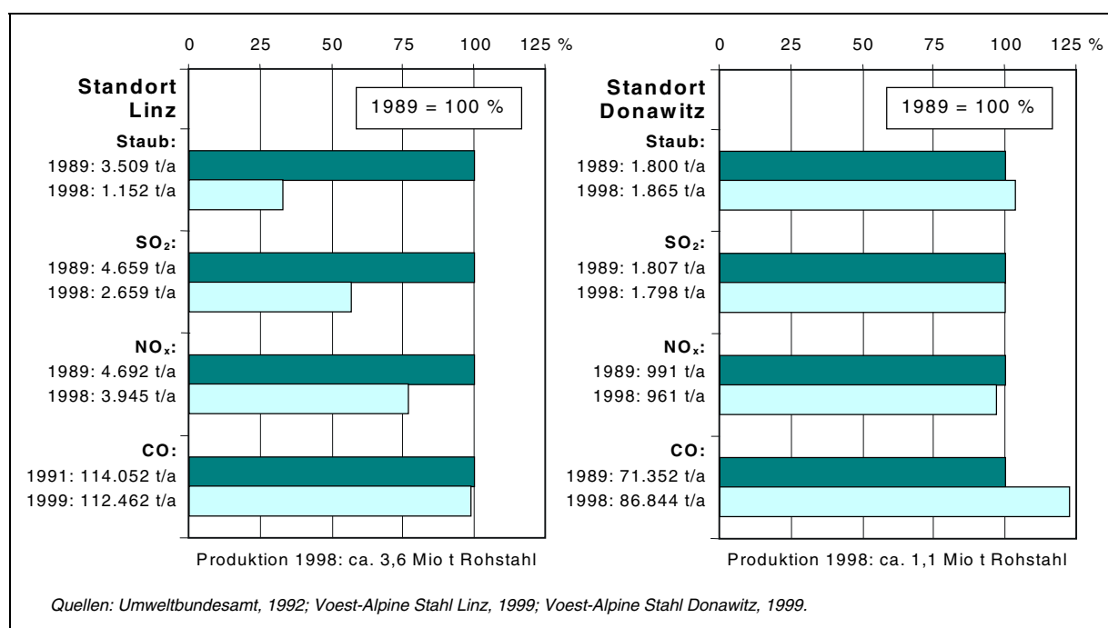
Abb. 8: Emissionen ausgewählter Luftschadstoffe bei der Herstellung von Roheisen und Stahl an den Standorten Linz bzw. Donawitz in den Jahren 1989 und 1998.
