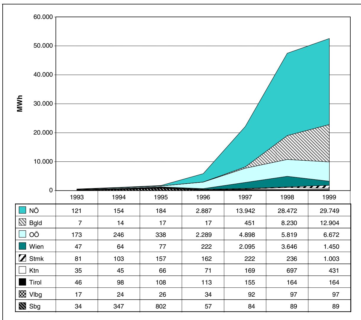
Abb. 8: Elektrische Energie aus Windkraft und Photovoltaik 1993-1999 nach Bundesländern.
