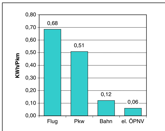
Abb. 7: Vergleich der Energieeffizienz der Verkehrsmittel im Personenverkehr in Kilowattstunden je Personenkilometer für das Jahr 1999.
