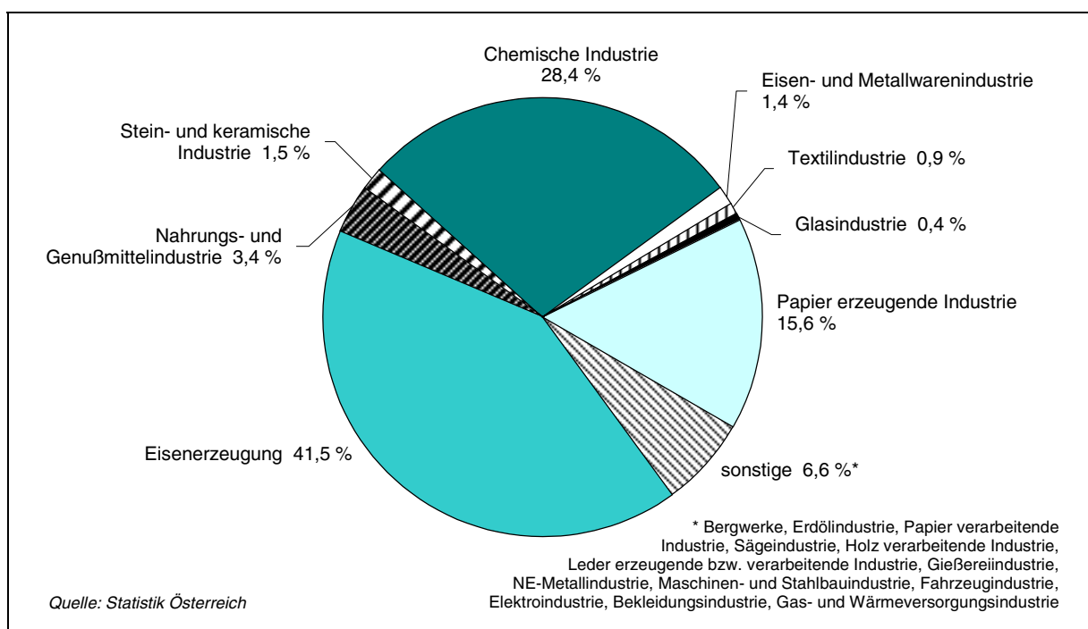
Abb. 7: Wasserverbrauch nach Fachverbänden im Jahr 1994.
