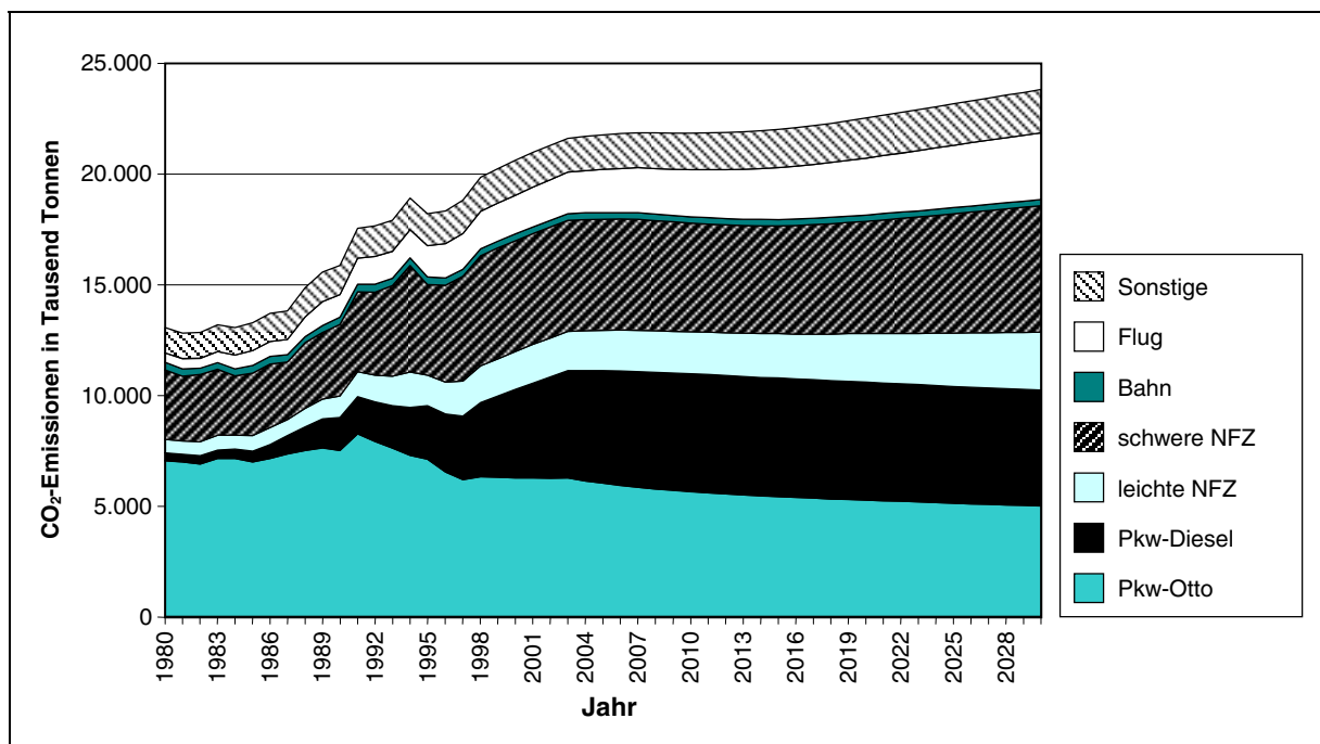
Abb. 21: Entwicklung der CO 2 -Emissionen nach Fahrzeugkategorie 1980-2030.
