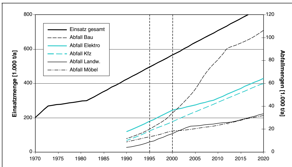
Abb. 16: Voraussichtliche Entwicklung der Nichtverpackungs-Kunststoffabfallmengen auf Basis einer Lebensdauerrechnung. Für die Einsatzmengen gilt die linke Werteskala, für die Abfallmengen die rechte Werteskala.
