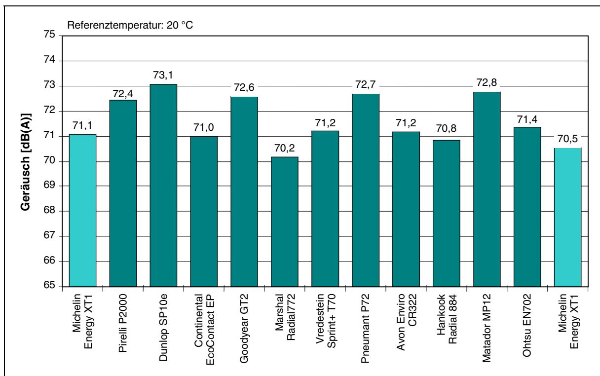
Abb. 6a: Schallpegel von Reifen verschiedener Erzeugung, gemessen nach Vorschlag zur Richtlinie 92/23/EWG. Reifen: 175/70 R 13 82T.
