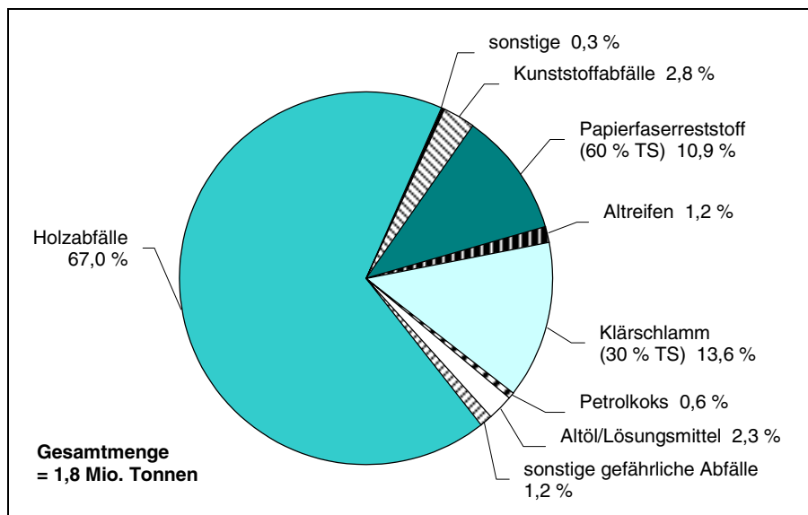
Abb. 13: Abfallmitverbrennung nach Abfallarten, Stand: 1998.
