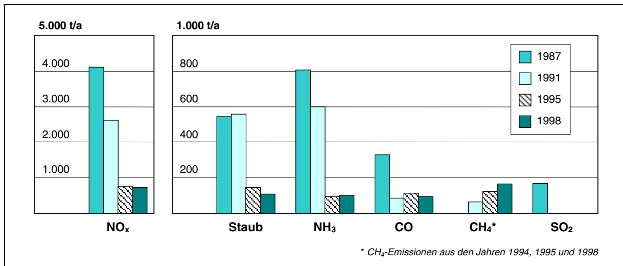
Abb. 12: Entwicklung ausgewählter Luftschadstoffemissionen aus der Herstellung von Grundchemikalien und Düngemitteln eines Betriebes am Standort Linz.
