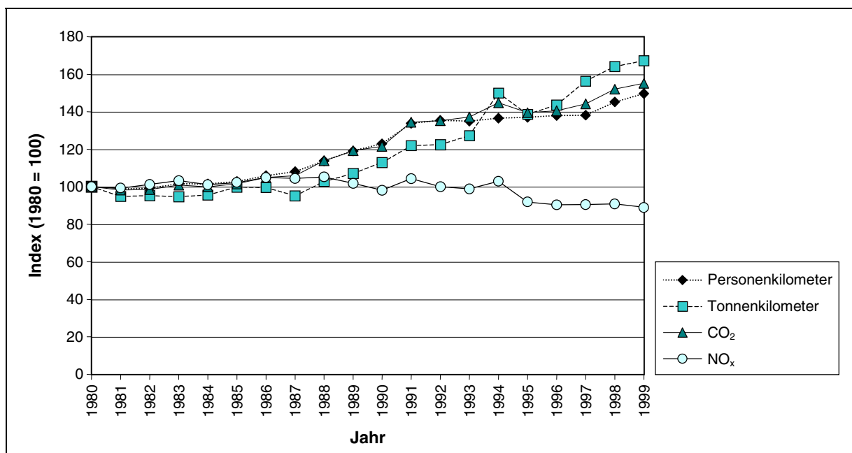
Abb. A: Entwicklung der Transportleistung im Güter- und im Personenverkehr sowie der CO 2 - und NO x -Emissionen von 1980-1999.
