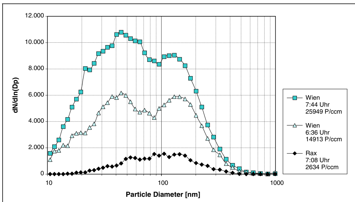
Abb. 24: Vergleich der Größenverteilung von Feinpartikelmessungen in Wien Währing und auf der Rax.
