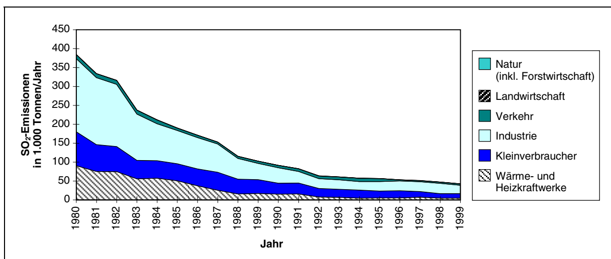
Abb. 16: Luftschadstoffemissionen an SO 2 in Österreich von 1980-1999.
