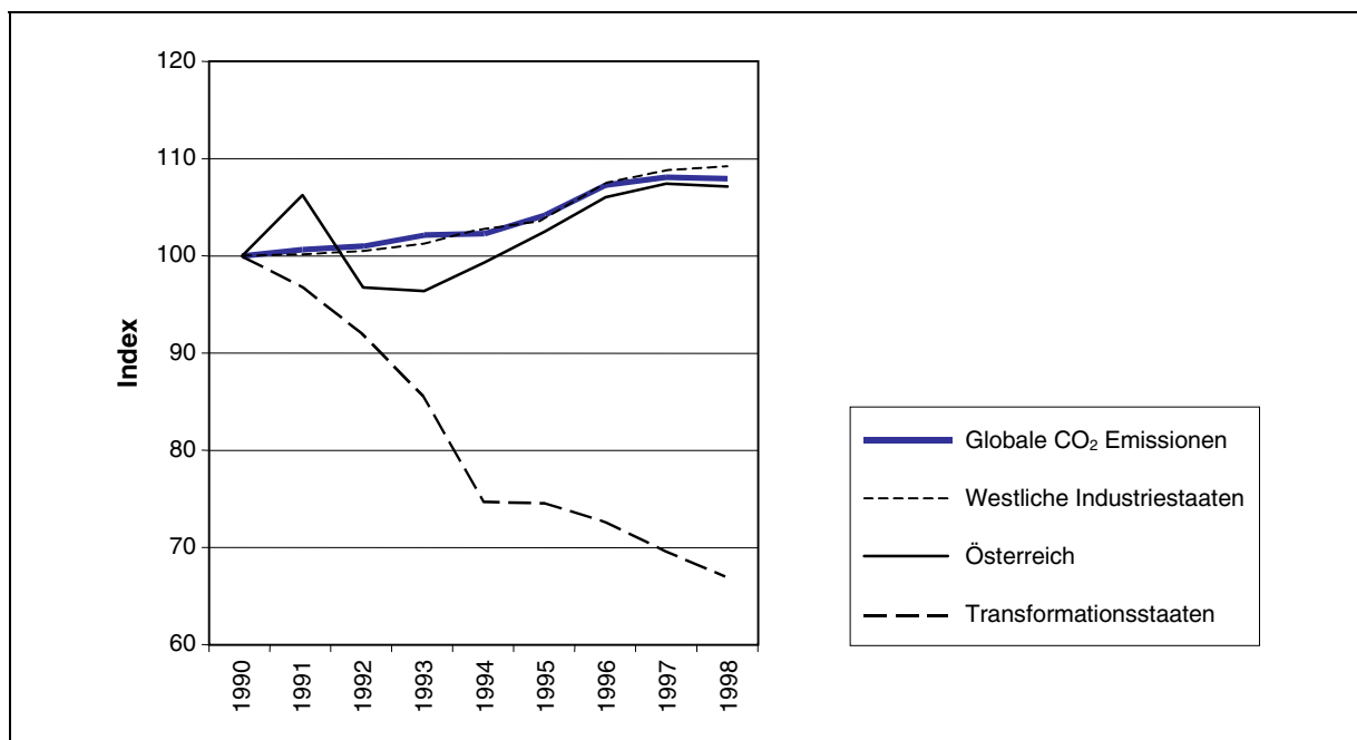
Abb. A: CO 2 -Emissionen global, der westlichen Industriestaaten, der Transformationsstaaten und Österreichs.
