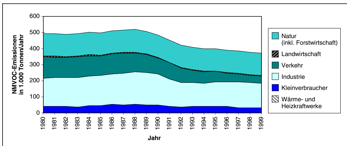
Abb. 7: Luftschadstoffemissionen an NMVOC in Österreich von 1980-1999.
