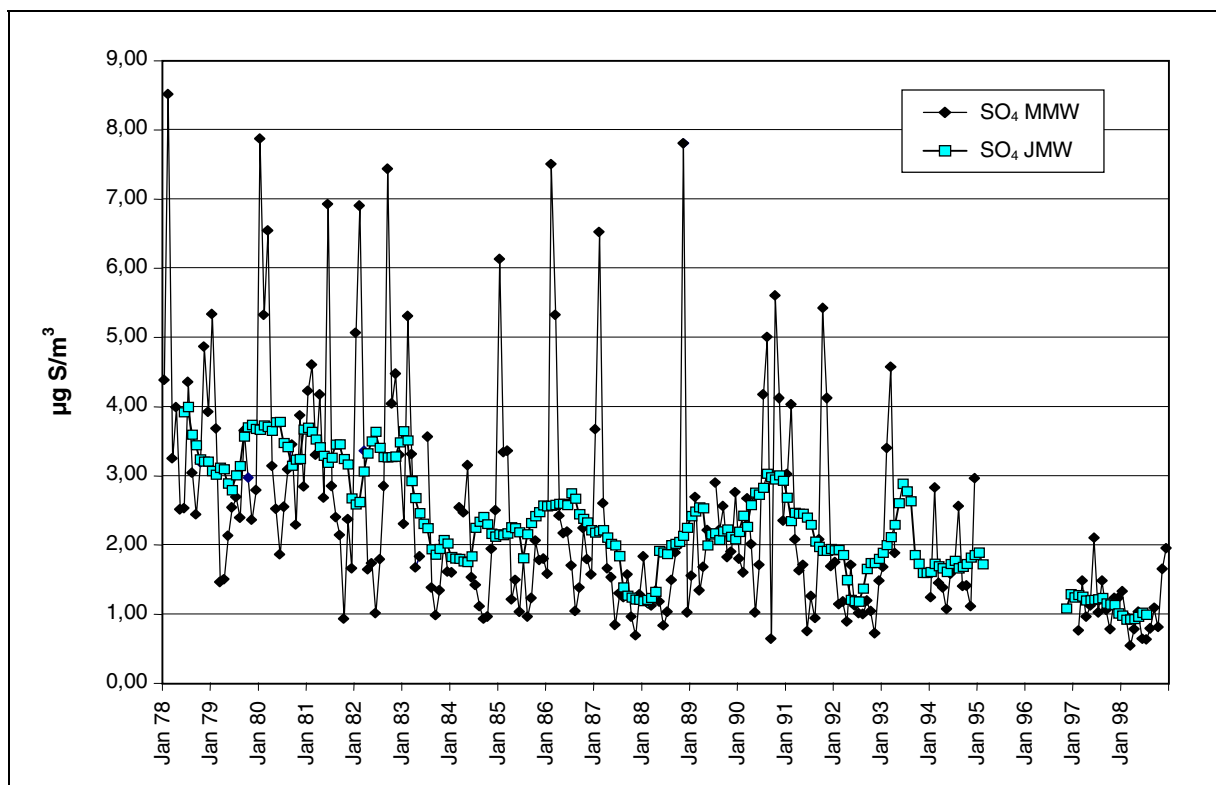
Abb. 5: Verlauf der Monatsmittelwerte bzw. des gleitenden Jahresmittelwertes der partikelgebundenen Sulfatkonzentration in Illmitz.
