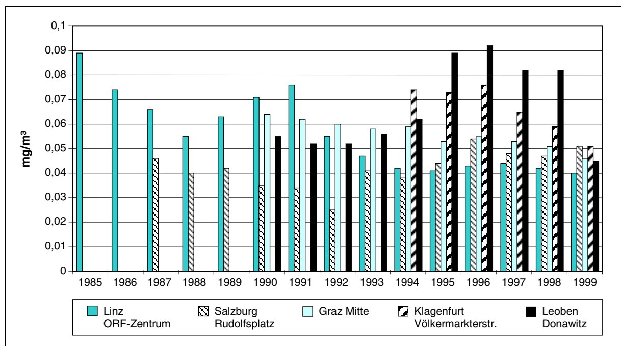
Abb. 4: Jahresmittelwert der Gesamtschwebestaubkonzentration an ausgesuchten Messstellen.
