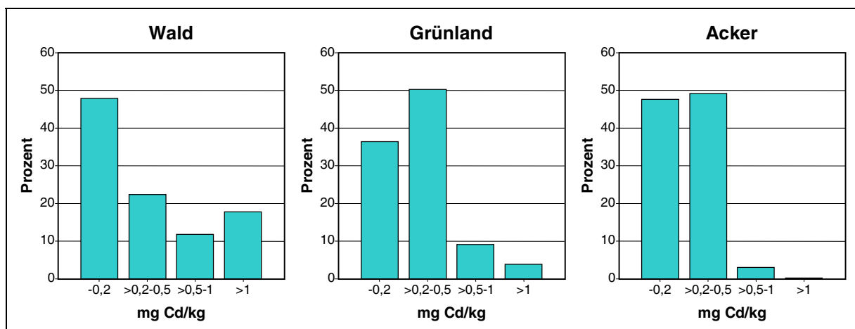
Abb. 5: Häufigkeitsverteilung (%) von Kadmium in den Oberböden (0-20cm) nach Bewertungsklassen in Wald, Grünland und Acker.
