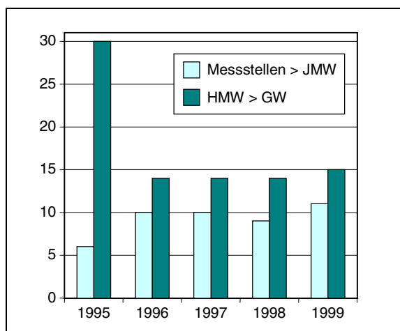
Abb. 15: Anzahl der Messstellen mit Überschreitungen des HMW von 0,20 \text{ mg}/\text{m}^3 bzw. des JMW von 0,040 \text{ } \mu\text{g}/\text{m}^3 in Österreich von 1995-1999.
