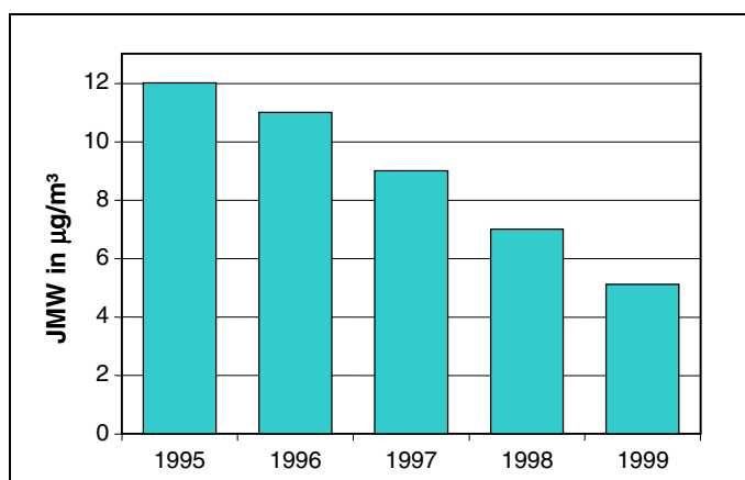
Abb. 27: Entwicklung des Jahresmittelwertes Benzol an dem Salzburger Standort Rudolfsplatz.
