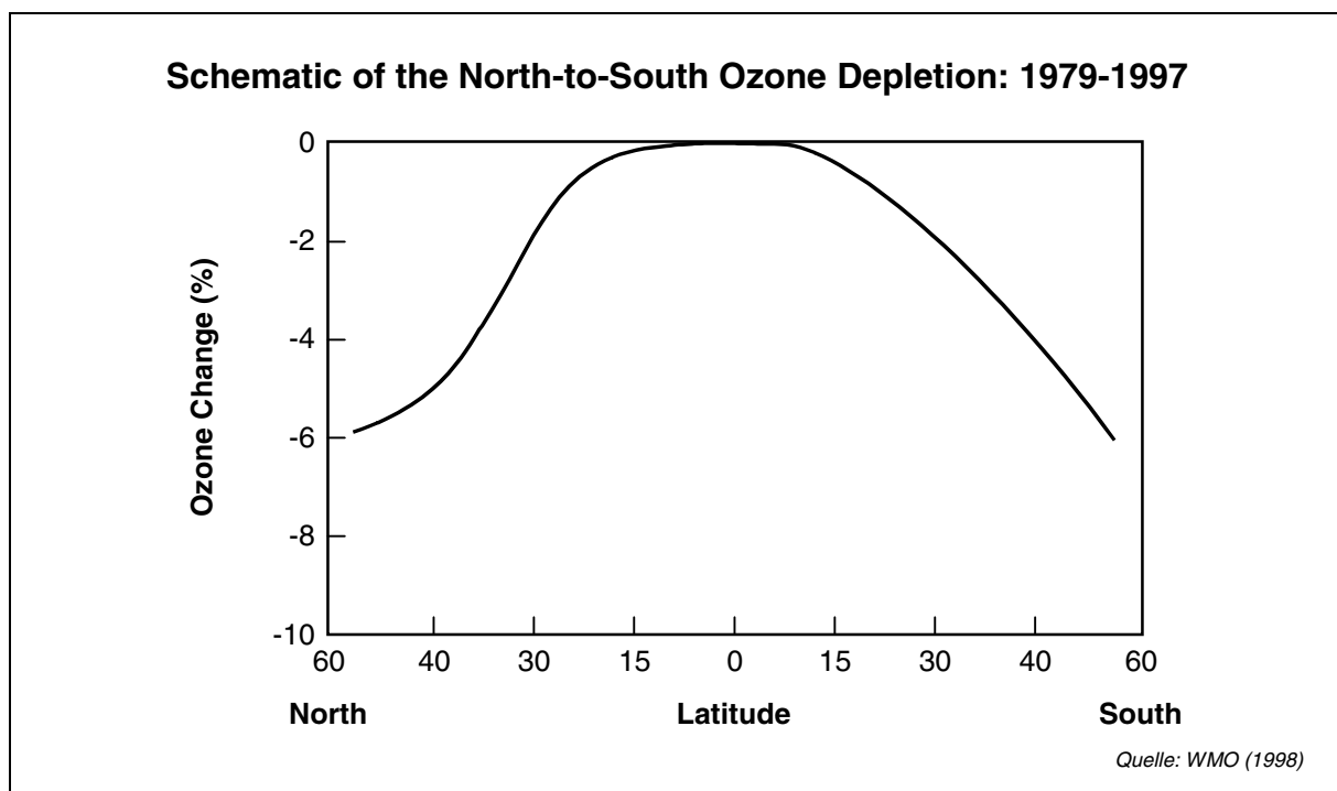
Abb. 2: Schematische Darstellung der Ausdünnung der Ozonschicht nach Breitengraden (1979-1997).
