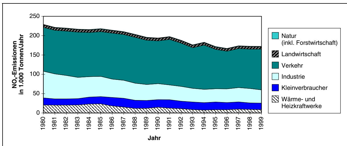
Abb. 8: Luftschadstoffemissionen an NO x in Österreich von 1980-1999.
