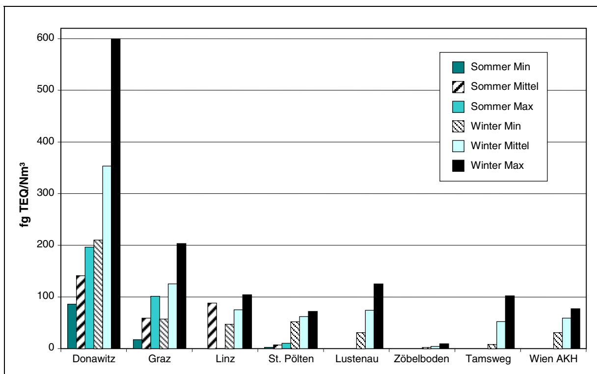
Abb. 29: Dioxinkonzentrationen in fg TEQ/Nm³ an ausgesuchten Standorten; Linz, Graz, Donawitz und St. Pölten: Winter 97/98 sowie Sommer 98. Lustenau, Zöbelboden, Tamsweg und AKH/Wien: Winter 98/99.
