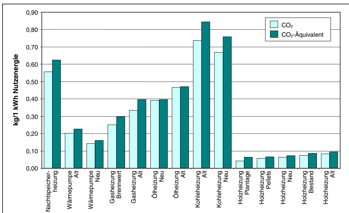
Abb. 13: Treibhausgasbilanz von Heizsystemen.
