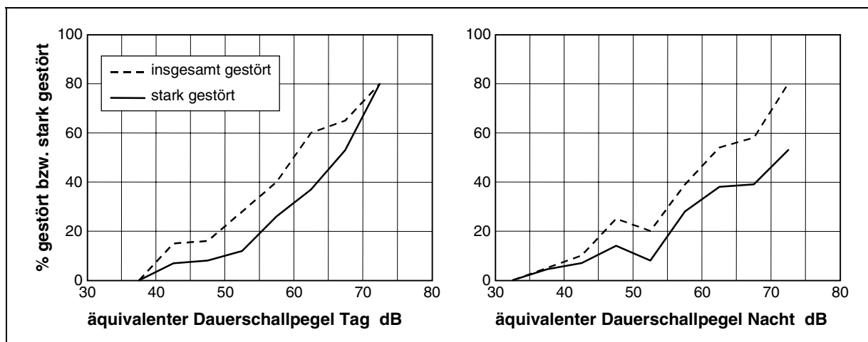
Abb. 2: Statistischer Zusammenhang zwischen dem Schallpegel und der Störwirkung von Schienenverkehrslärm.
