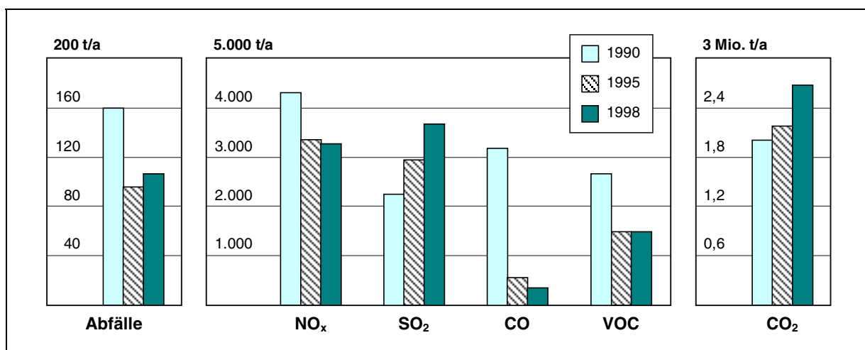
Abb. 11: Entwicklung der bei der Raffination von Erdöl in Schwechat auftretenden Emissionen ausgewählter Luftschadstoffe Staub, NO x , SO 2 , CO, VOC und CO 2 (nach: ECKER & WINTER, 2000).
