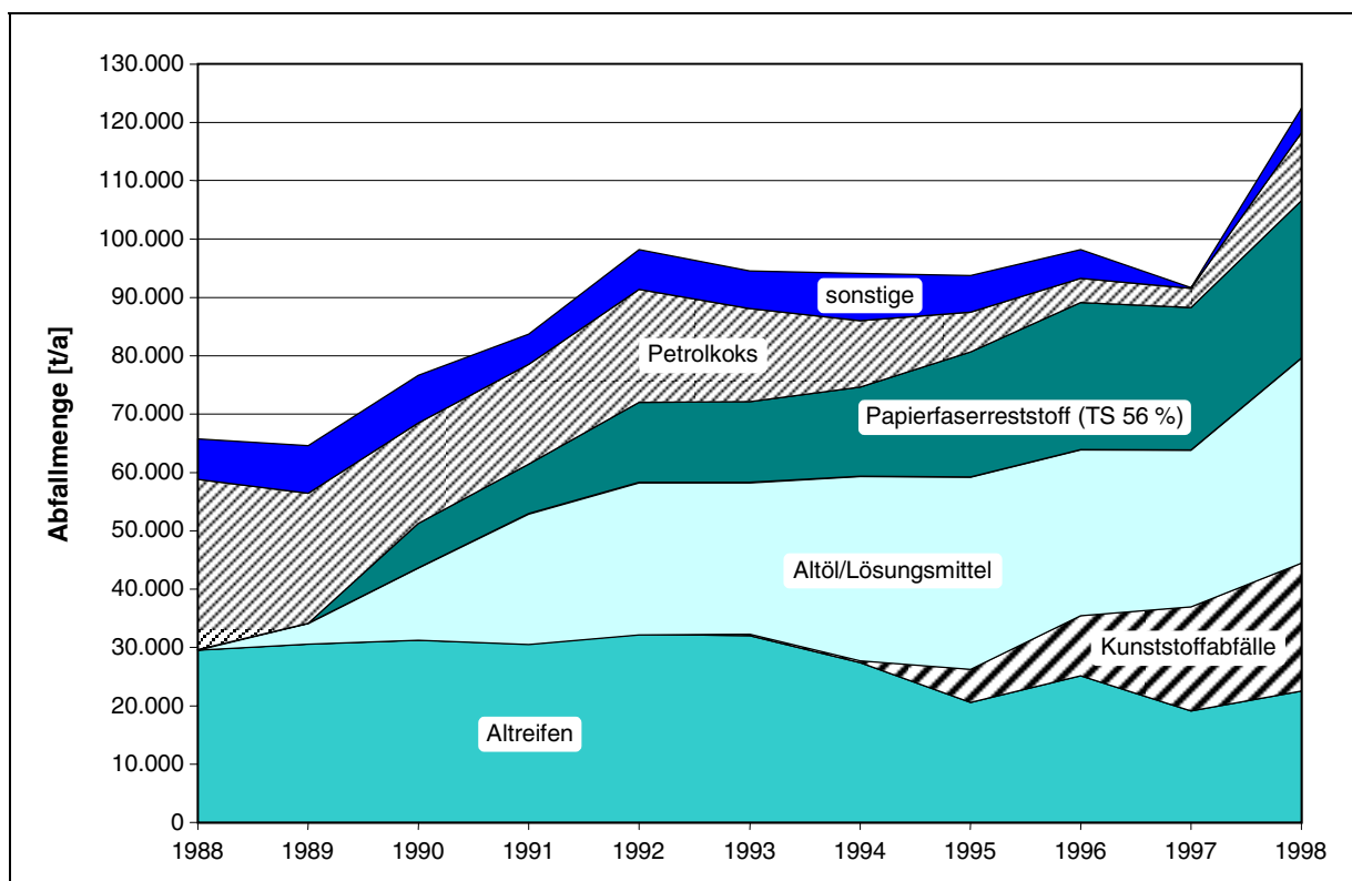
Abb. 15: Abfalleinsatz in der österreichischen Zementindustrie seit 1988, Darstellung der Gesamtentwicklung.
