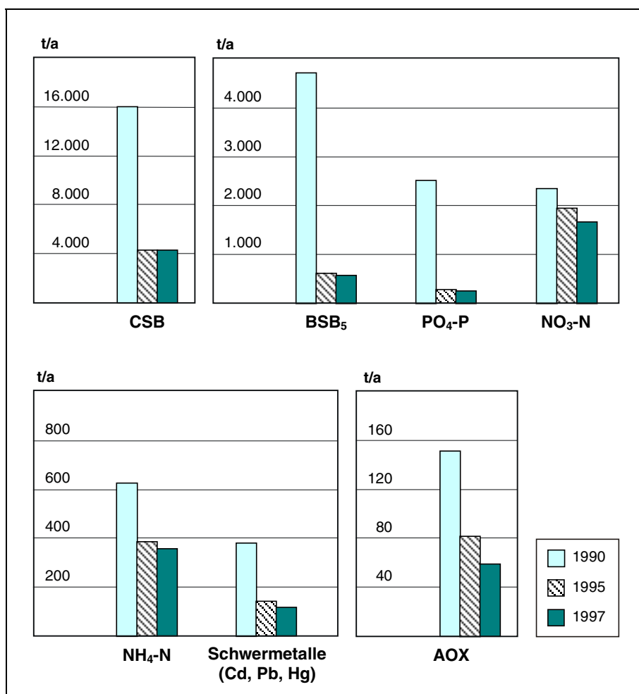
Abb. 13: Entwicklung der Abwasseremissionen in der chemischen Industrie.
