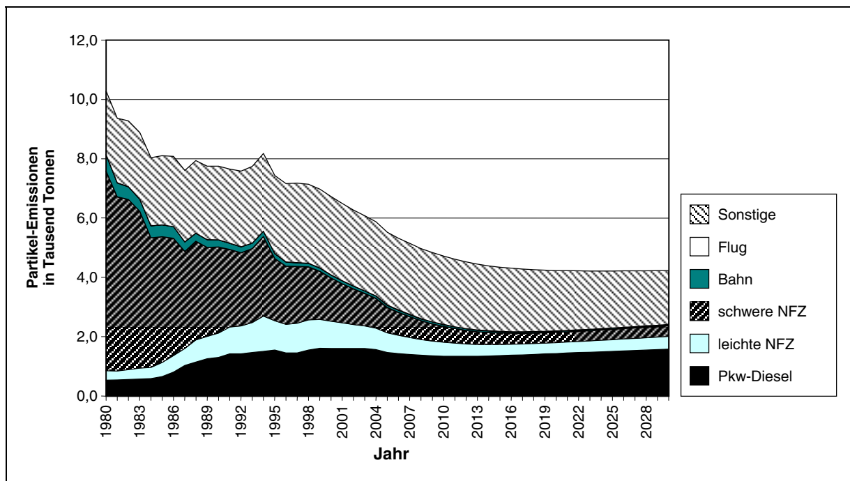
Abb. 23: Entwicklung der Partikel-Emissionen nach Fahrzeugkategorie 1980-2030.
