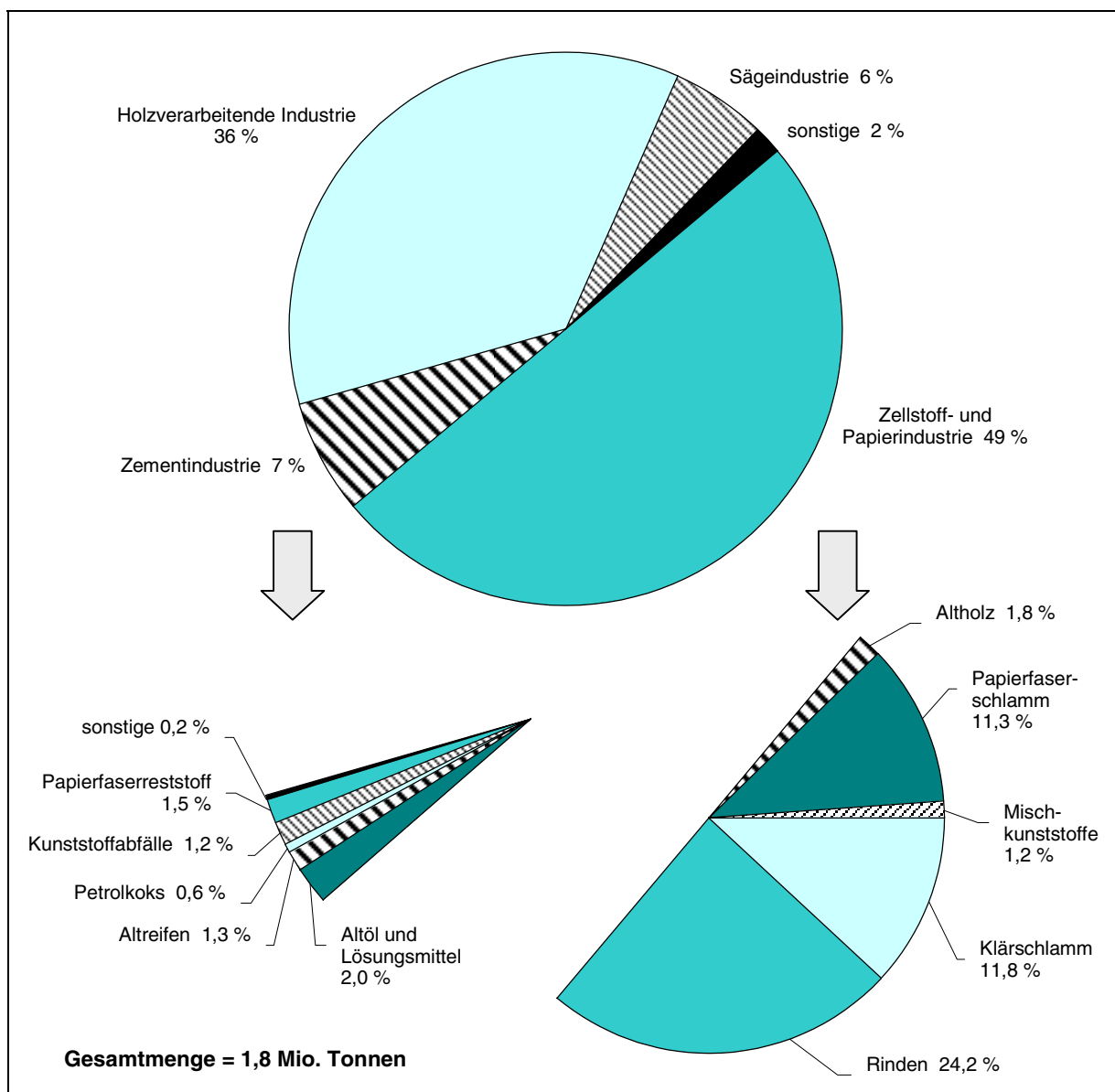
Abb. 12: Abfallmitverbrennung in industriellen Feuerungsanlagen, gegliedert nach Branchen bzw. Abfallarten (Stand: 1998).
