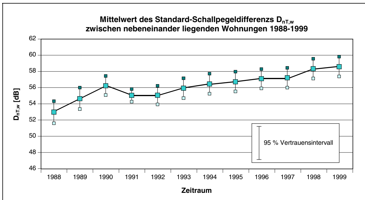
Abb. 8b: Ergebnisse der bauakustischen Messungen in Wohnhäusern im Land Oberösterreich (Luftschallschutz).
