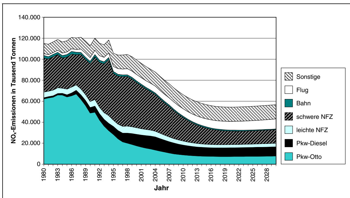
Abb. 22: Entwicklung der NO x -Emissionen nach Fahrzeugkategorie 1980-2030.
