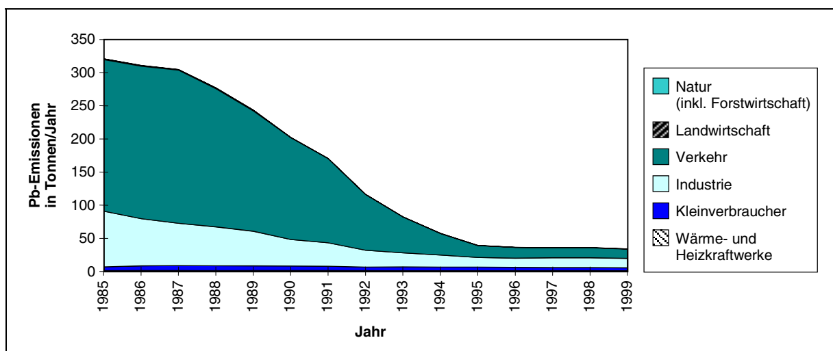
Abb. 26: Luftschadstoffemissionen an Blei in Österreich von 1985-1999.
