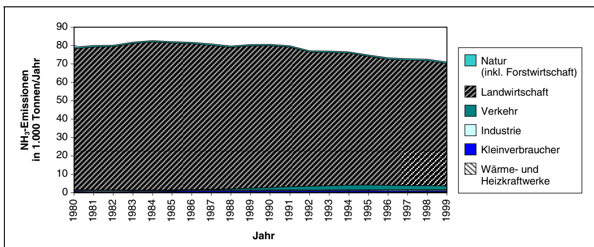
Abb. 32: Luftschadstoffemissionen an \text{NH}_3 in Österreich von 1980-1999.
