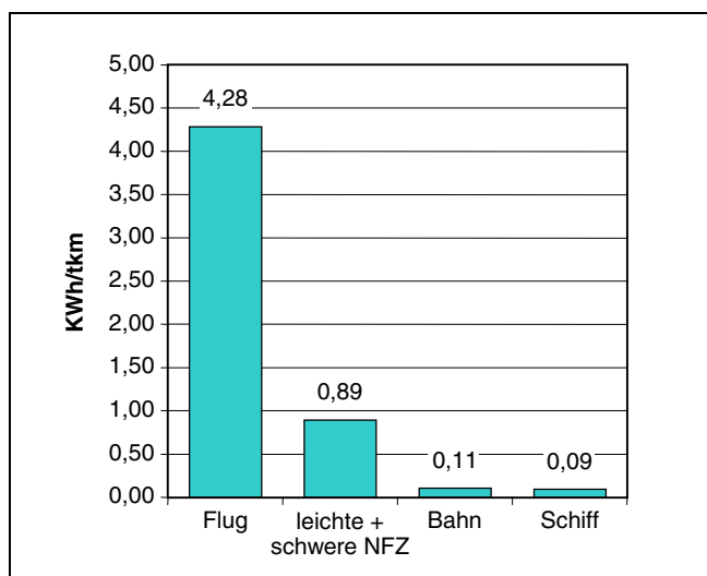
Abb. 8: Vergleich der Energieeffizienz der Verkehrsmittel im Güterverkehr in Kilowattstunden je Tonnenkilometer für das Jahr 1999.
