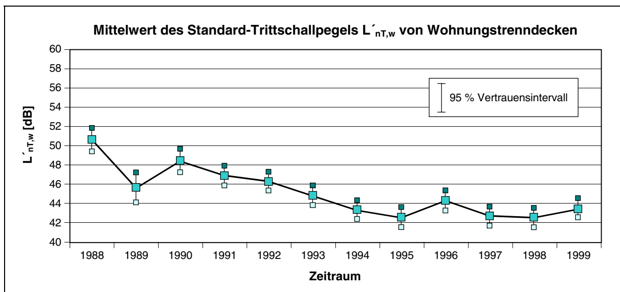
Abb. 8a: Ergebnisse der bauakustischen Messungen in Wohnhäusern im Land Oberösterreich (Trittschallschutz) von 1988-1999. Das Vertrauensintervall ist ein Maß für die Unsicherheit.
