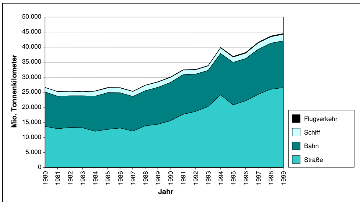
Abb. 5: Transportleistung aufgeschlüsselt nach Verkehrsträgern für die Jahre 1980-1999 in Millionen Tonnenkilometern.
