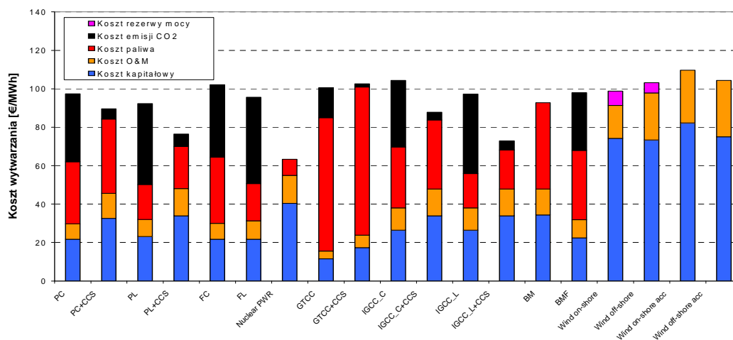
Rys. 4.10. Porównanie uśrednionych kosztów wytwarzania energii elektrycznej i ich struktury dla źródeł przewidzianych do uruchomienia około 2030 r. Źródło – Analiza ARE wykonana w 2009r. na zlecenie MG
