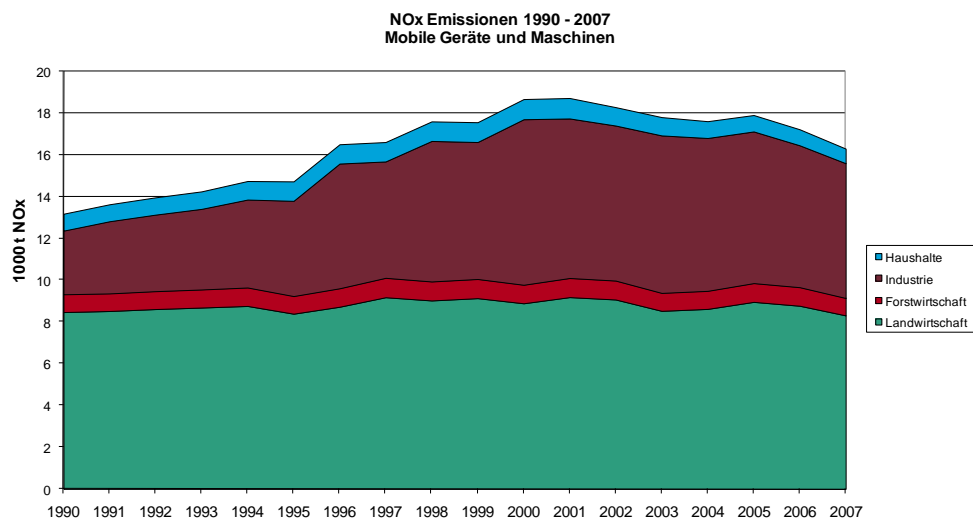
Abbildung 1: NOx Emissionen Mobile Geräte und Maschinen
