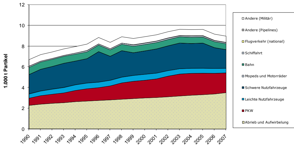
Partikelemissionen 1990 - 2007 Verkehrssektor
