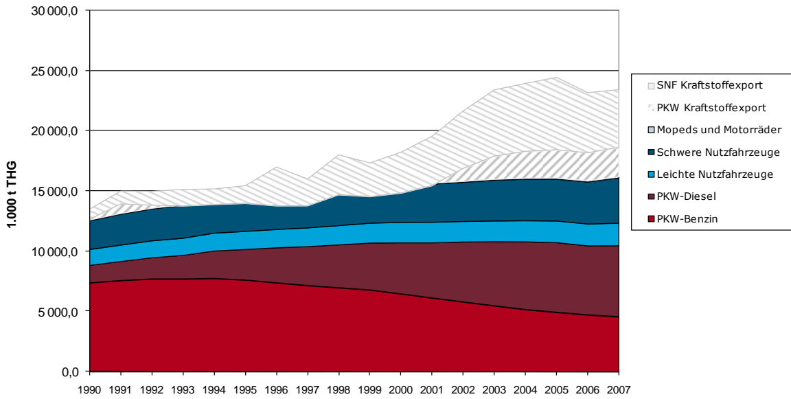
THG Emissionen 1990 - 2007 Straßenverkehr
