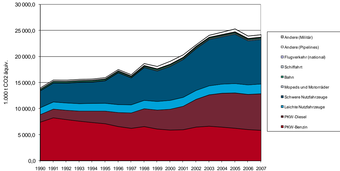
THG Emissionen 1990 - 2007 Verkehrssektor
