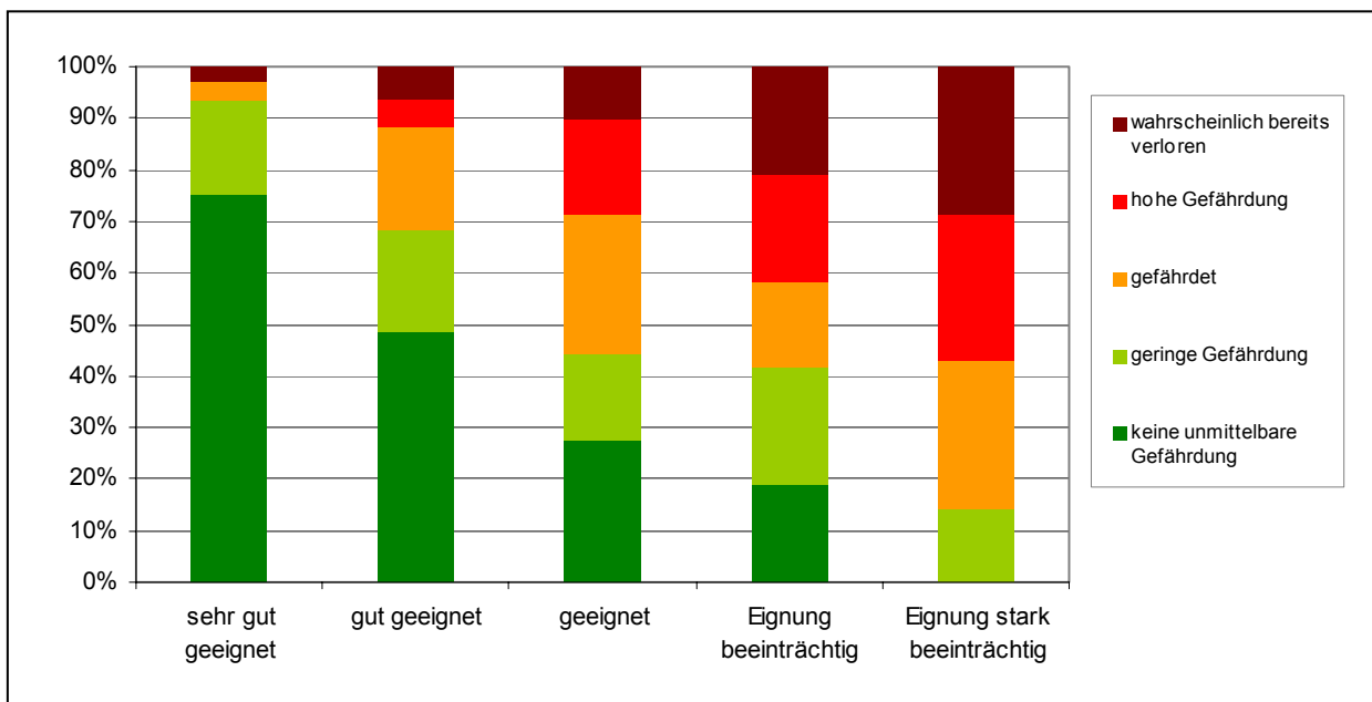
Abbildung 20: Querungszonen mit hoher Eignung sind seltener von absehbaren Zerstörungen bedroht, als Zonen, die aufgrund ihrer Strukturausstattung oder Lage weniger geeignet erscheinen. Dargestellt sind Anteile der Gefährdungsklassen (in Prozent) pro Eignungskategorie.
