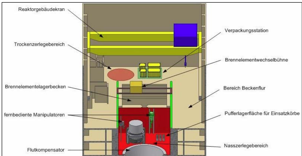
Abbildung 7: Prinzipdarstellung, Schnittbild Reaktordruckbehälter mit Einbauten, geplanter Abbaubereich in Phase 1
