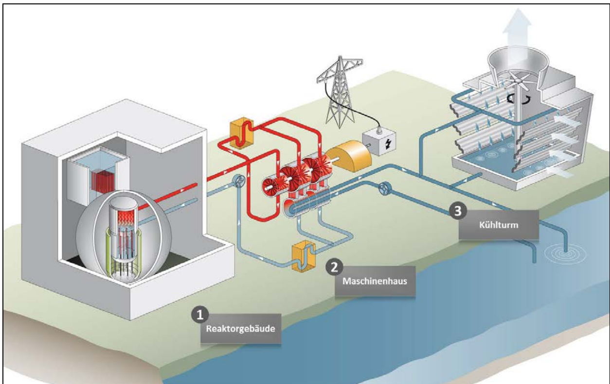
Abbildung 3: Prinzipielle Darstellung der Arbeitsweise eines Siedewasserreaktors
