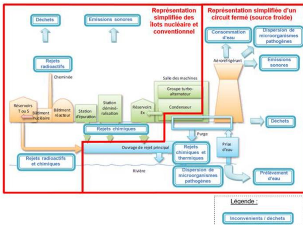
Figure 33 : Schéma type d'une centrale nucléaire de type REP en bord de fleuve refroidie en circuit dit « fermé »
