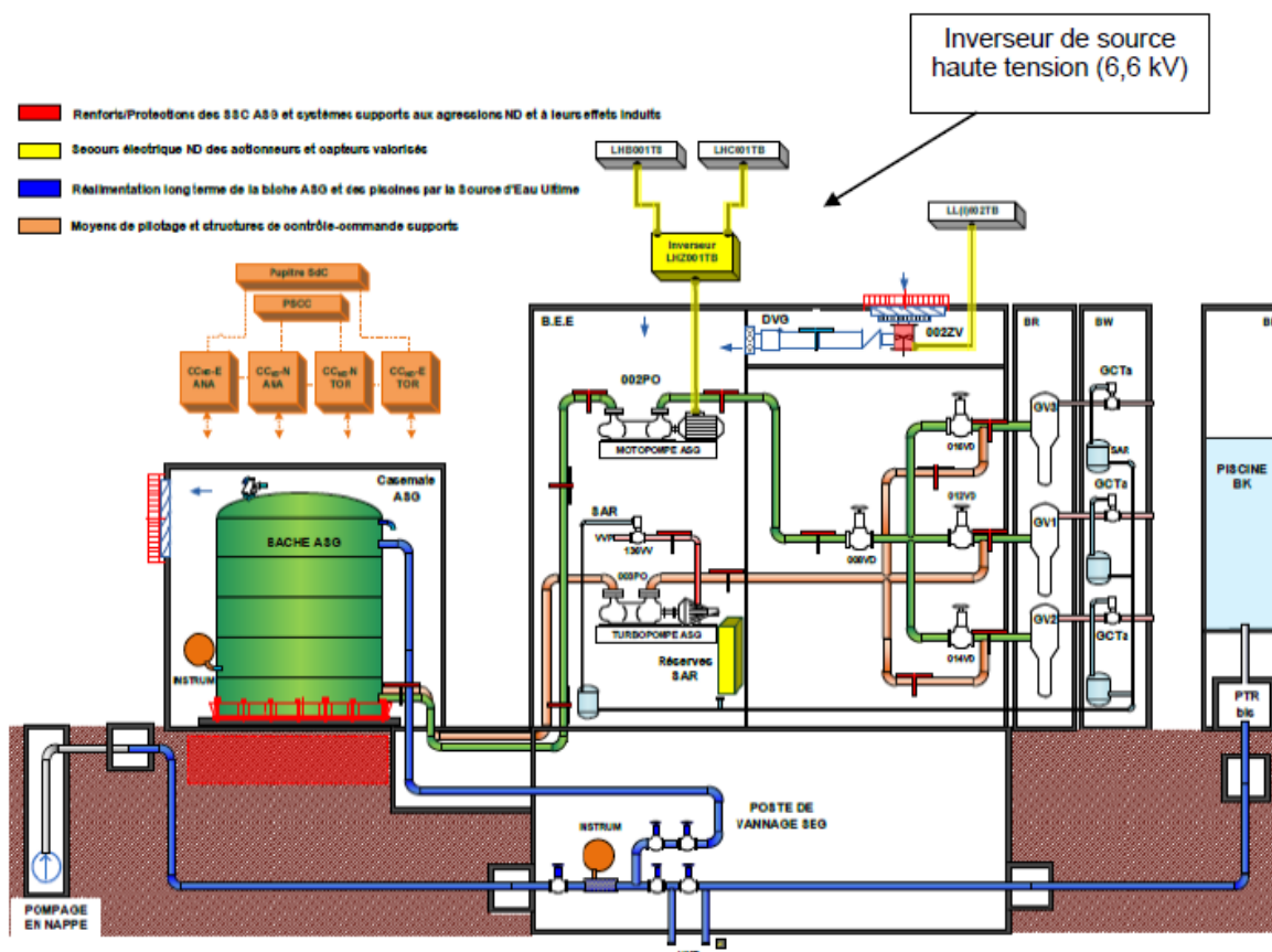
Schéma de principe de la disposition ASG-ND
