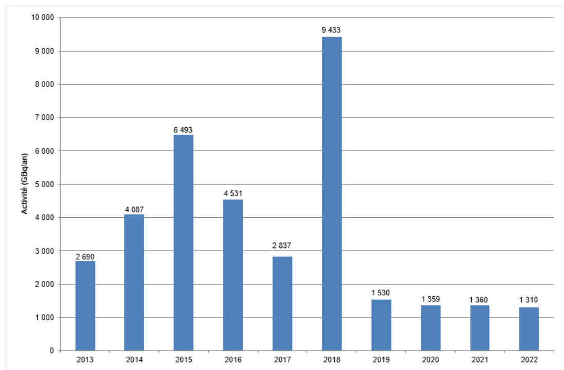
Activité en gaz rares rejetée à l'atmosphère sur la période 2013-2022 de la centrale de Gravelines
