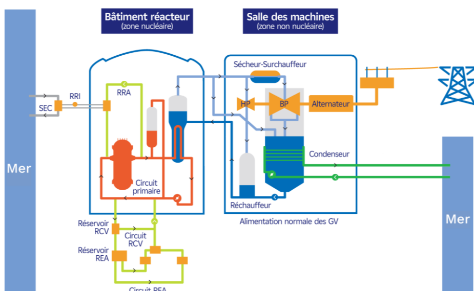
Figure 1. Réacteur en fonctionnement normal : principaux circuits
