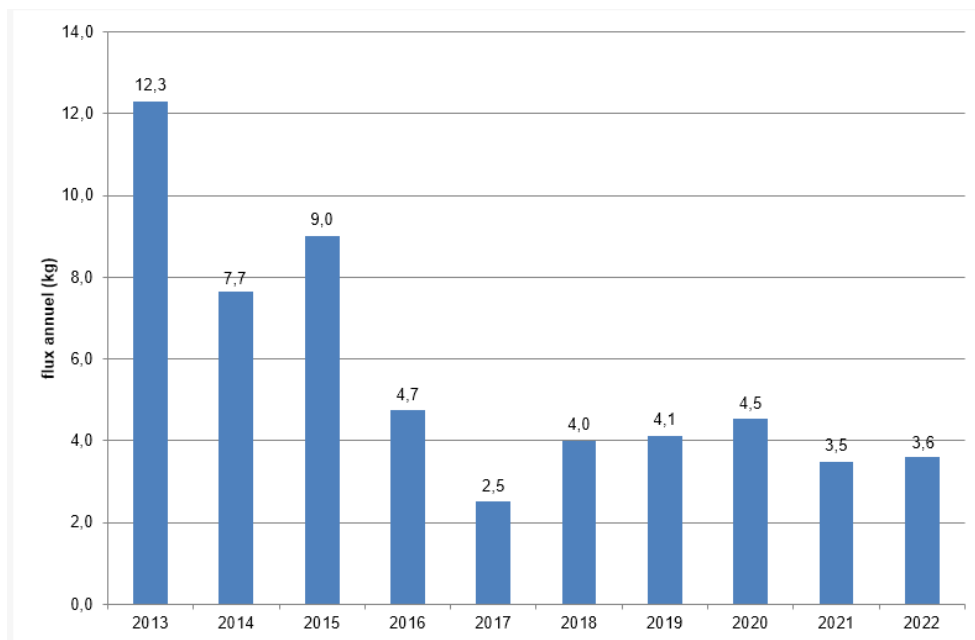
Rejets annuels d'hydrazine sur la période 2013 – 2022 de la centrale de Gravelines
