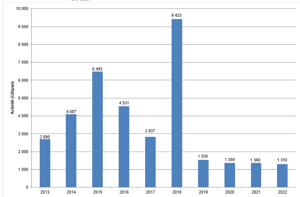
Figure 4 : Activité en gaz rares rejetée à l'atmosphère du CNPE de Gravelines sur la période 2013 – 2022
