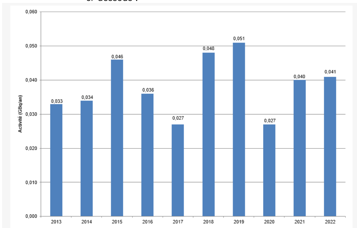
Figure 6 : Activité en iode rejetée dans les effluents liquides du CNPE de Gravelines sur la période 2013 - 2022
