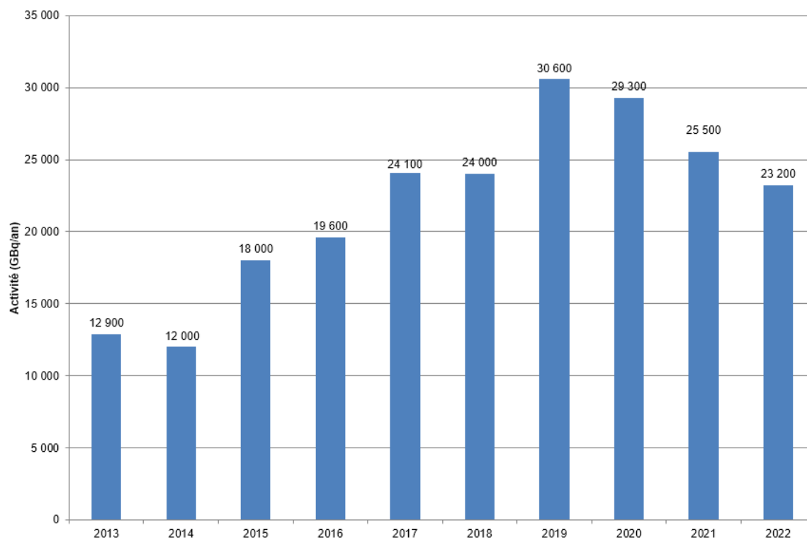
Figure 9 : Rejets annuels d'acide borique sur la période 2013 – 2022 du CNPE de Gravelines
