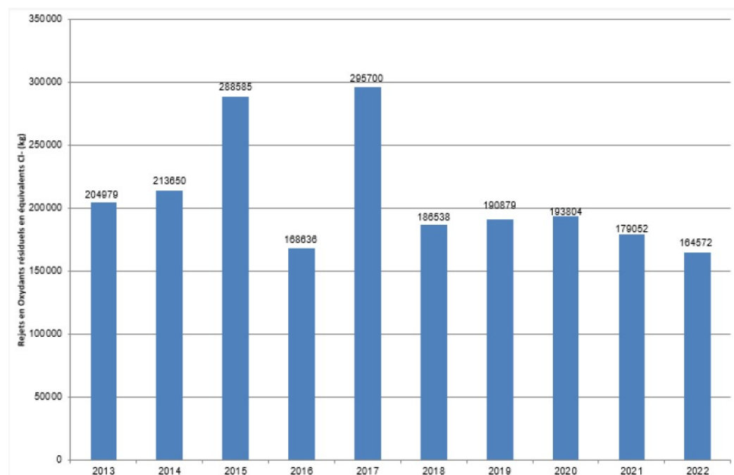
Figure 16 : Rejets annuels d'ORT issus de l'électrochloration du CNPE de Gravelines sur la période 2013 – 2022
