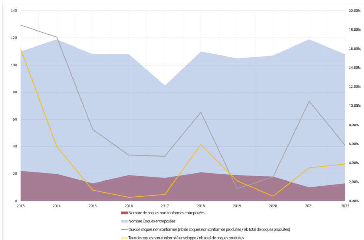
Figure 30 : Évolution de la qualité des coques déchets produites sur le CNPE de Gravelines sur la période 2013-2022
