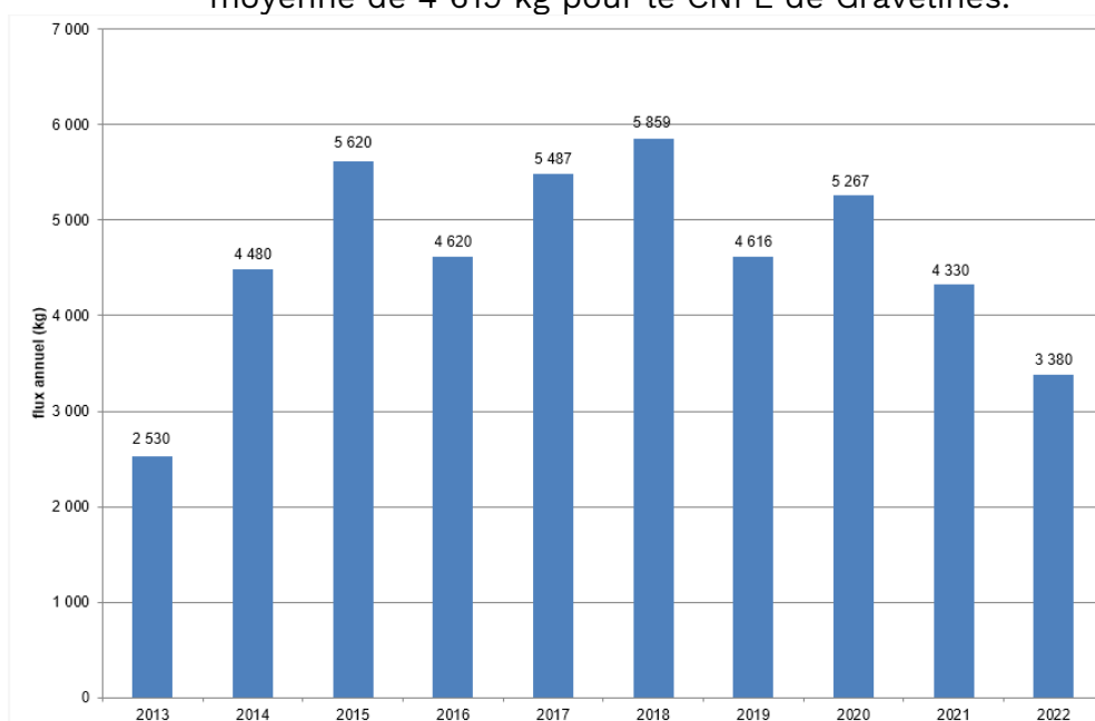
Figure 13 : Rejets annuels d'azote total sur la période 2013 – 2022 du CNPE de Gravelines
