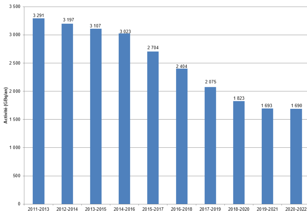
Figure 3 : Activité en tritium rejetée à l'atmosphère, moyenne sur 3 années glissantes sur la période 2013 – 2022, du CNPE de Gravelines
