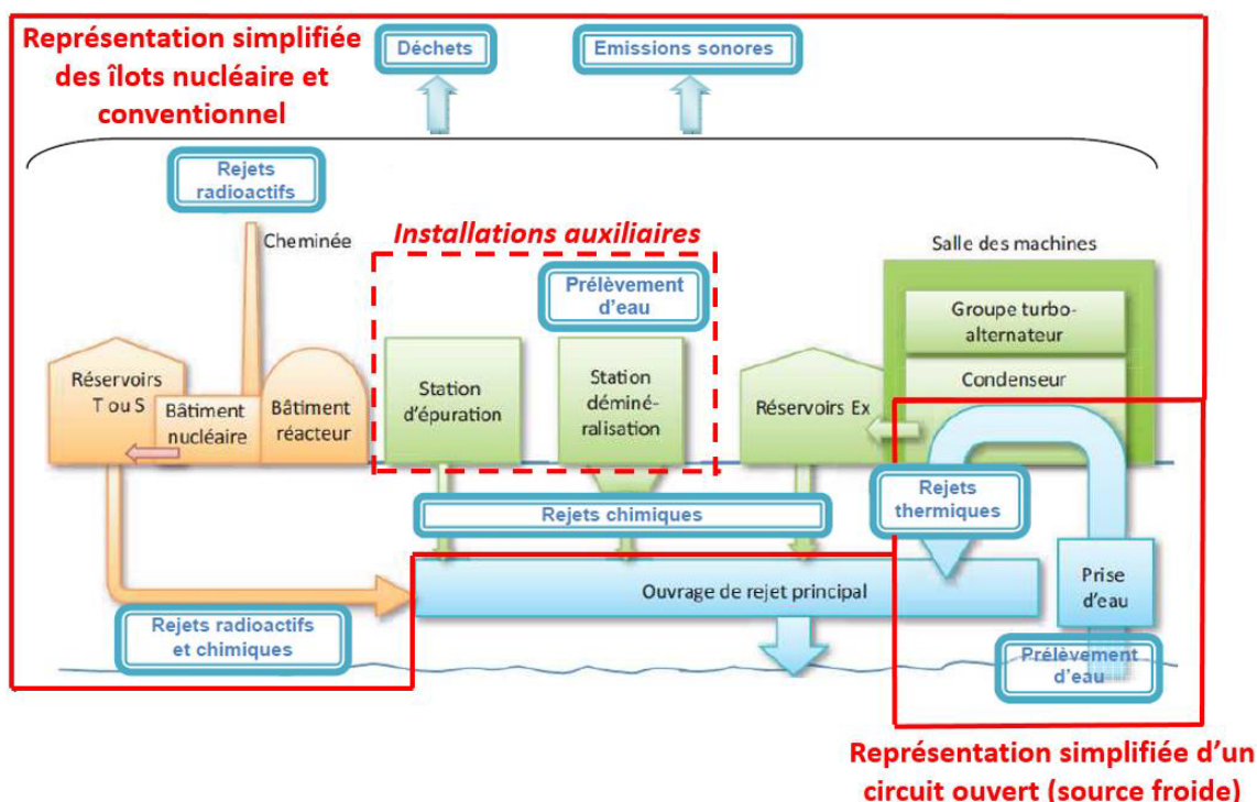
Figure 29 : Présentation schématique des îlots nucléaire et conventionnel et de la source froide ainsi que des inconvénients associés (CNPE en bord de mer, refroidi en circuit ouvert)
