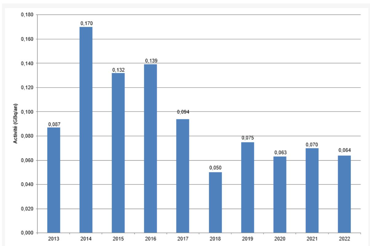
Figure 5 : Activité en iodes rejetée à l'atmosphère par le CNPE de Gravelines sur la période 2013 – 2022
