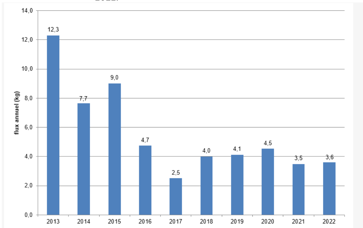
Figure 10 : Rejets annuels d'hydrazine sur la période 2013 – 2022 du CNPE de Gravelines
