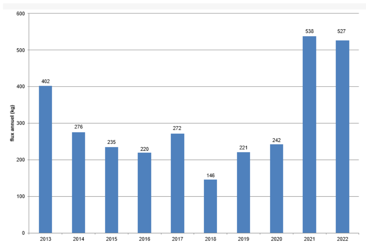
Figure 14 : Rejets annuels en phosphates du CNPE de Gravelines sur la période 2013 - 2022
