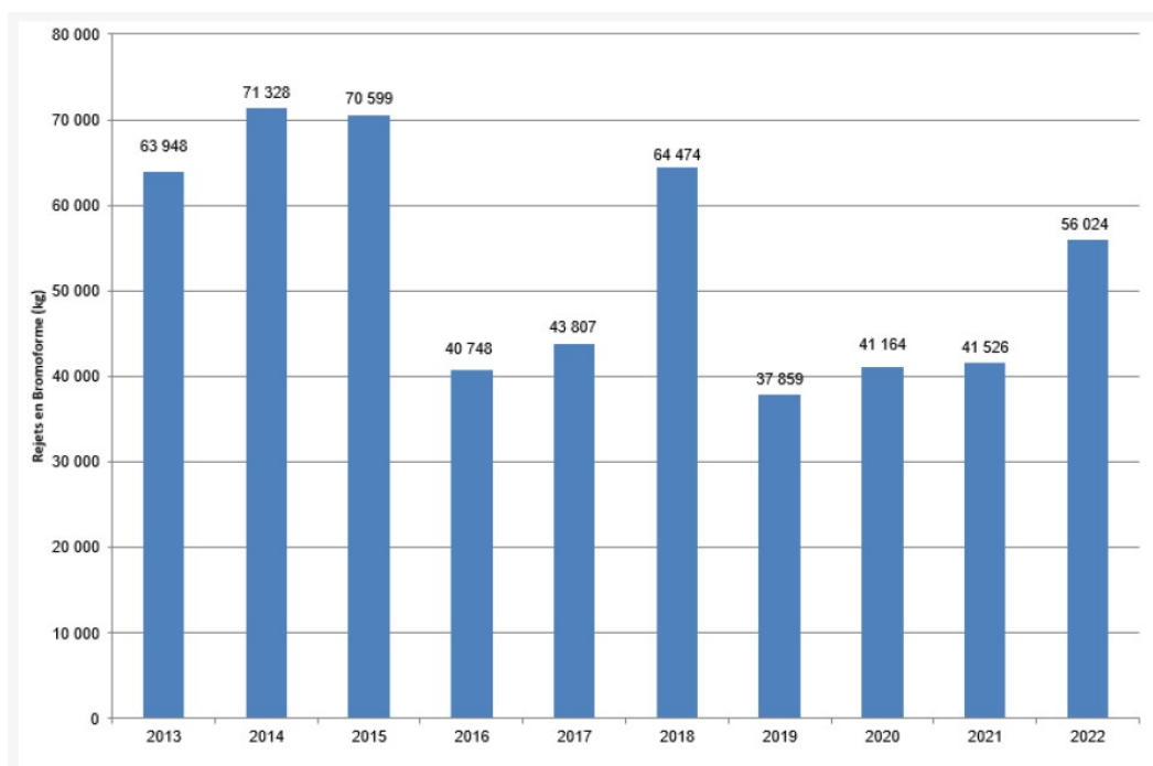
Figure 15 : Rejets annuels de bromoformes issus de l'électrochloration du CNPE de Gravelines sur la période 2013 – 2022
