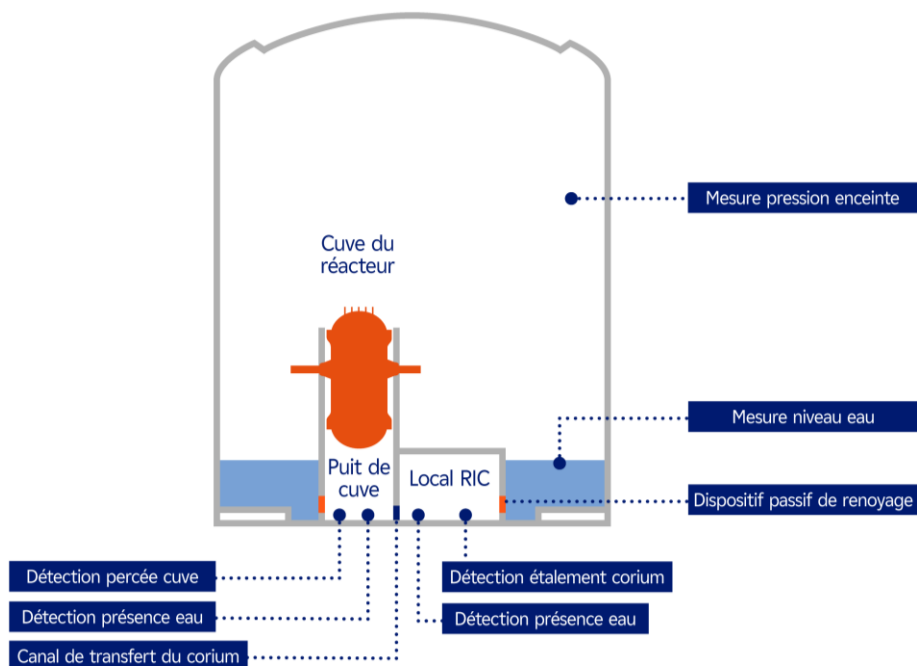
Figure 12. Illustration de la mesure de niveau d'eau dans les puits du bâtiment réacteur et de la détection de l'étalement du corium dans le local d'instrumentation du cœur (RIC)
