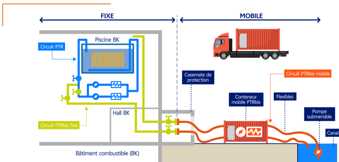
Figure 18. Appoint Noyau Dur par le haut de la piscine d'entreposage du combustible (représenté par la tuyauterie verte sur le schéma à droite de la piscine d'entreposage du combustible)
