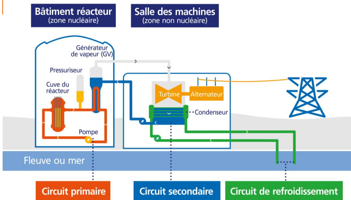
Figure 24. Principes de fonctionnement d'une centrale nucléaire
