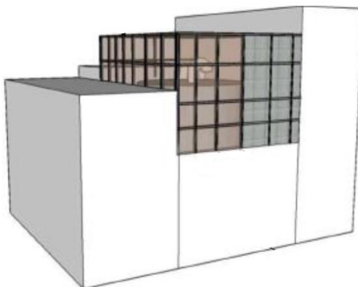
Figure 19. Protection contre la tornade « Noyau Dur » : photo de l'installation actuelle et illustration de la disposition proposée, de type « grilles renforcées », autour de la bâche PTR cylindrique.
