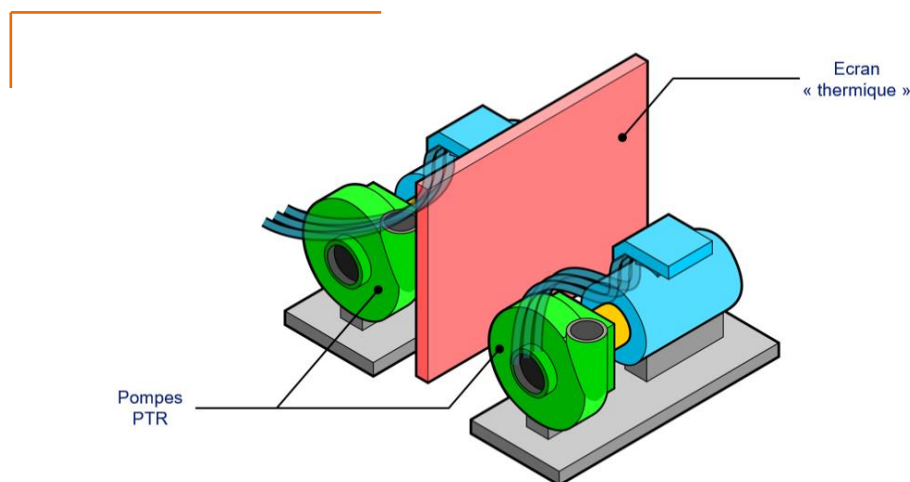
Figure 9. Installation d'un écran thermique entre les pompes du système de refroidissement de la piscine d'entreposage du combustible
