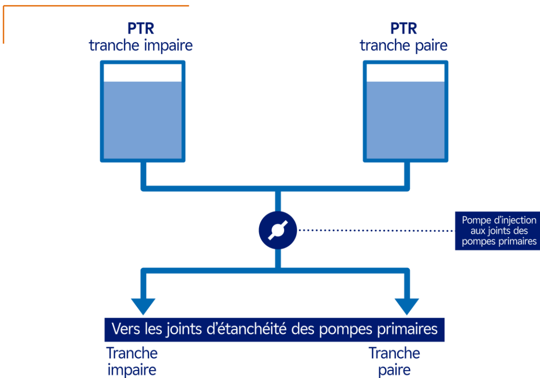
Figure 16. Configuration avant l'installation de la pompe d'injection aux joints « Noyau Dur » (PIJ-ND)
