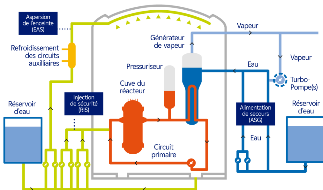
Figure 26. Systèmes de sauvegarde : 3 principaux circuits (ASG, RIS, EAS)
