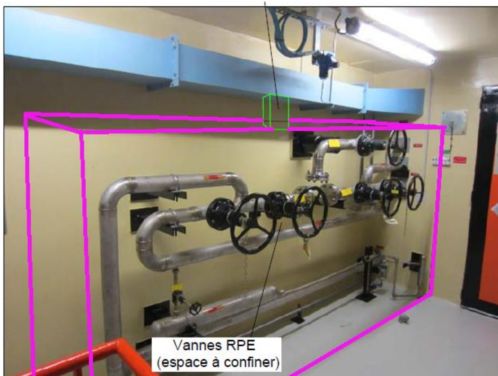
Figure 21. Création d'une enceinte ventilée raccordée à la filtration iode autour de certains équipements du système de collecte des effluents de l'îlot nucléaire (RPE) : photo du local et emplacement de la disposition
