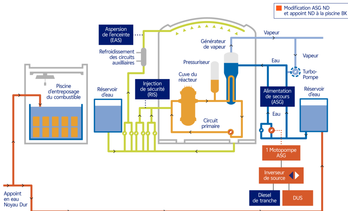
Figure 15. Schéma de principe de la disposition ASG-ND et appoint Noyau Dur aux piscines BR et BK
