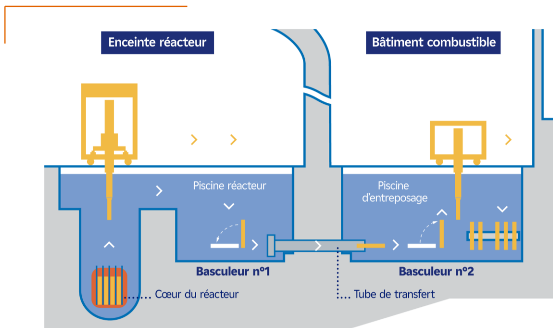
Figure 10. Piscine du bâtiment réacteur et piscine d'entreposage du combustible (illustration du transfert d'un assemblage de combustible du cœur du réacteur vers la piscine d'entreposage)
