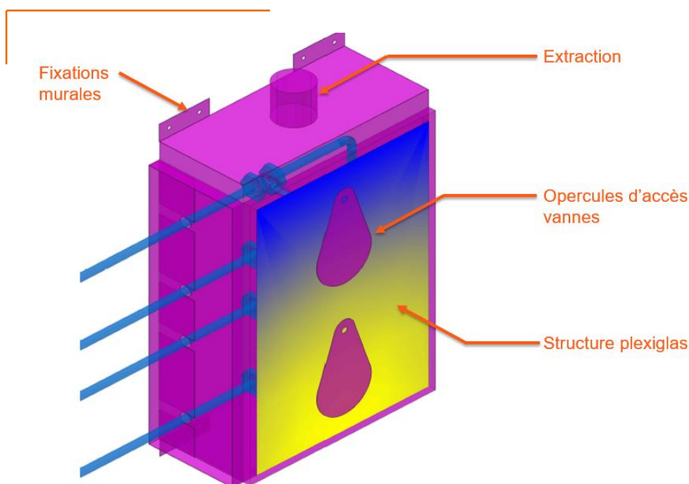
Figure 22. Création d'une enceinte ventilée raccordée à la filtration iode autour de certains équipements du système de collecte des effluents de l'îlot nucléaire (RPE) : illustration de la disposition
