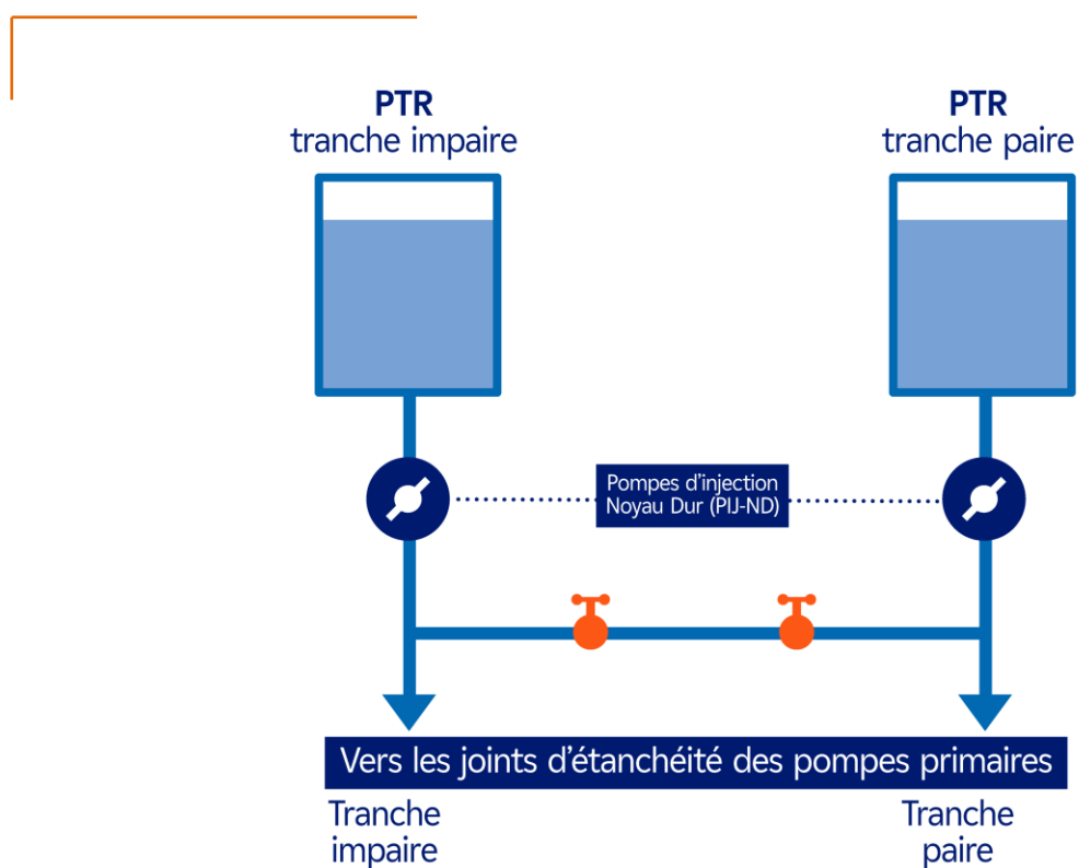
Figure 17. Configuration avec pompes d'injection aux joints « Noyau Dur » (PIJ-ND)
