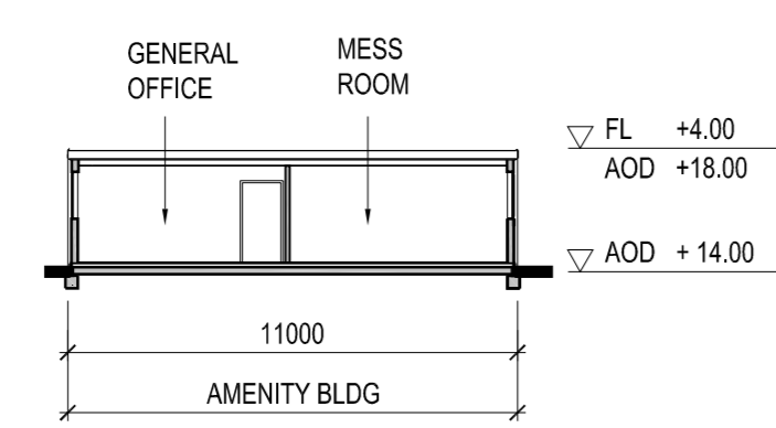
5 SECTION E/E SCALE 1:200
