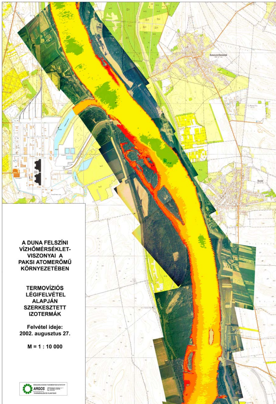
9. ábra A Duna felszíni vízhőmérséklet-viszonyai a Paksi Atomerőmű térségében a 2002. augusztus 27-i légifelvétel alapján
