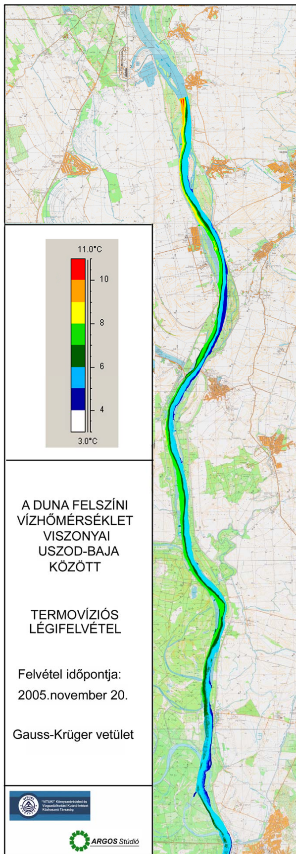
14. ábra A Duna felszíni vízhőmérséklet viszonyai Úszód-Baja között a 2005. november 20-i légifelvétel alapján
