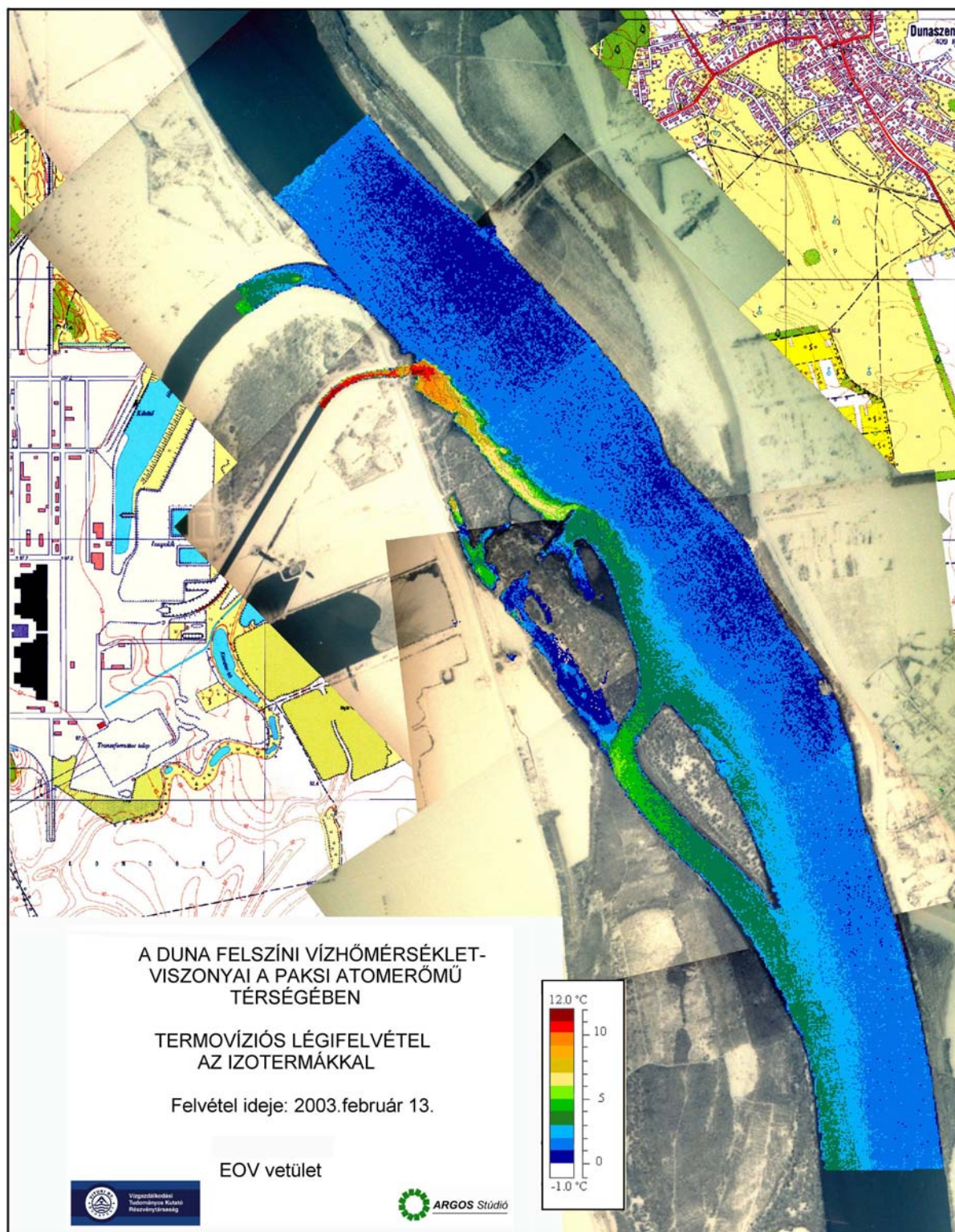
11. ábra A Duna felszíni hőképe a Paksi Atomerőmű térségében a 2003. február 13-i légifelvétel alapján
